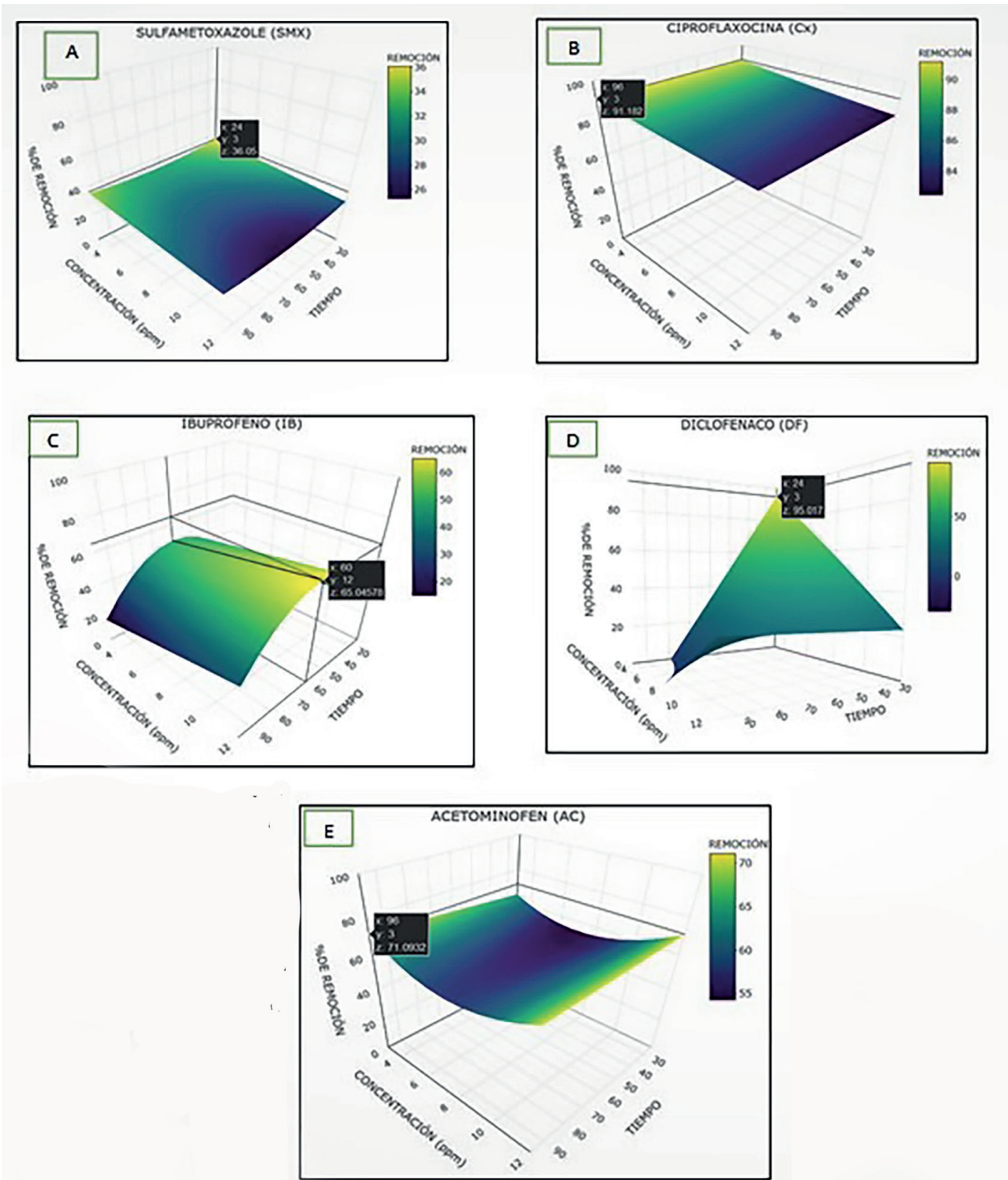
Figura 2. Resultados obtenidos con la técnica superficie de respuesta para la remoción con Eichhornia crassipes de los fármacos A) sulfametoxazol (SMX), B) ciprofloxacina (CX), C) ibuprofeno (IBU), D) diclofenaco (DF) y E) acetaminofén (AC) en medio acuoso.
